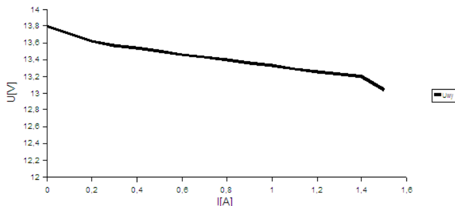
Rys. 4. Charakterystyka prądowo-napięciowa zasilacza.
