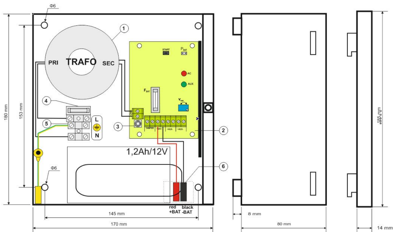
Rys.3. Widok zasilacza.
