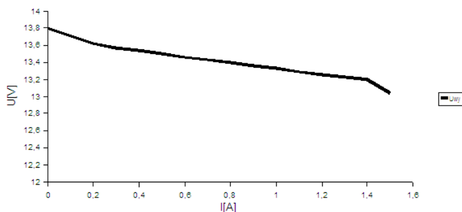
Rys. 4. Charakterystyka prądowo-napięciowa zasilacza.
