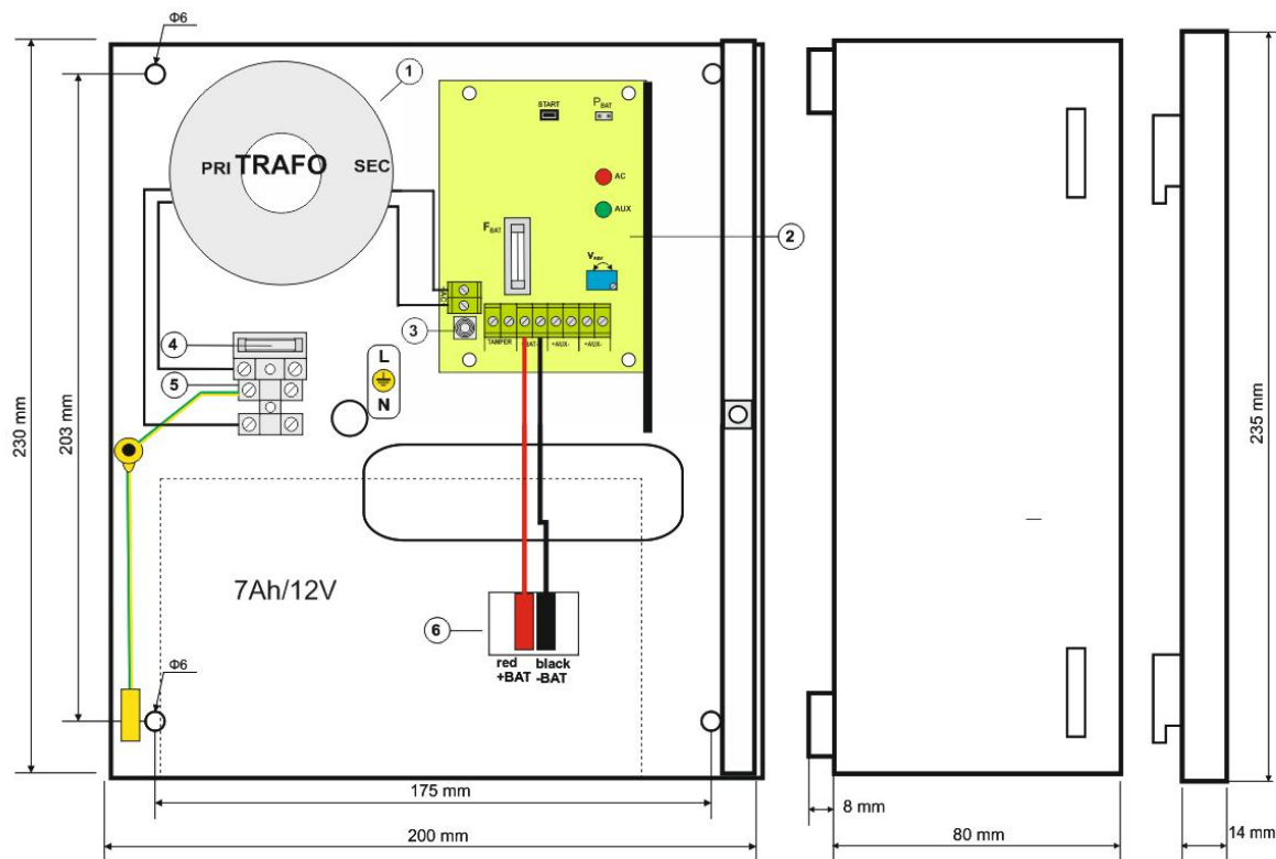
Rys.3. Widok zasilacza.
