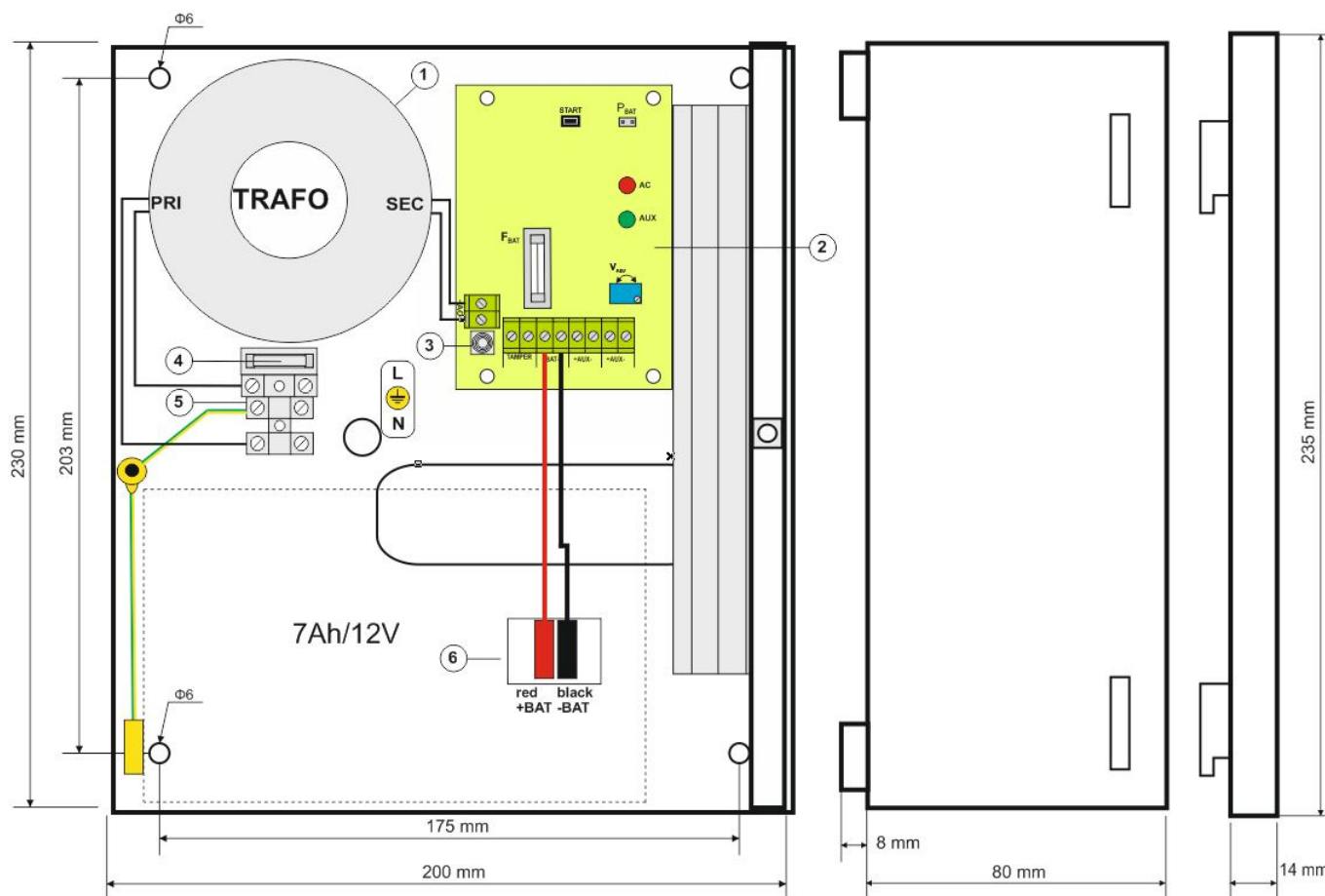
Rys.3. Widok zasilacza.
