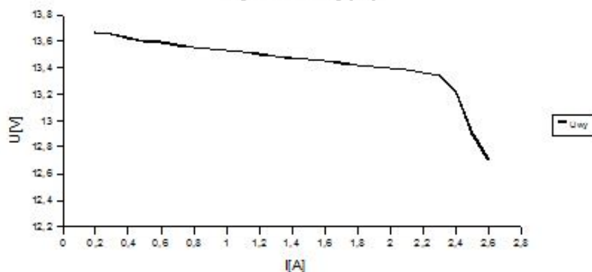
Rys. 4. Charakterystyka prądowo-napięciowa zasilacza.
