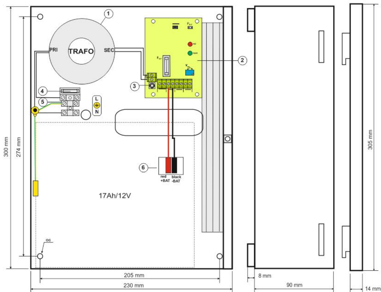
Rys.3. Widok zasilacza.
