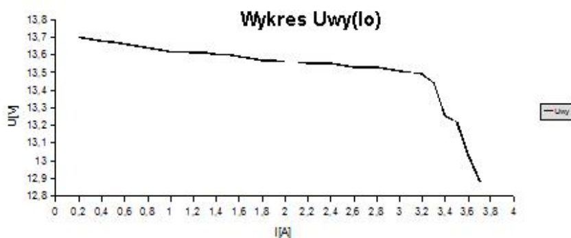
Rys. 4. Charakterystyka prądowo-napięciowa zasilacza.
