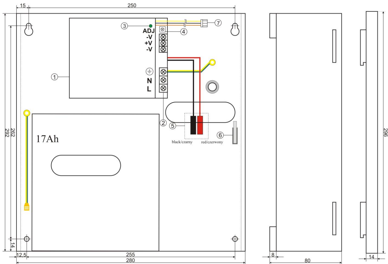
Rys.2. Widok zasilacza.
