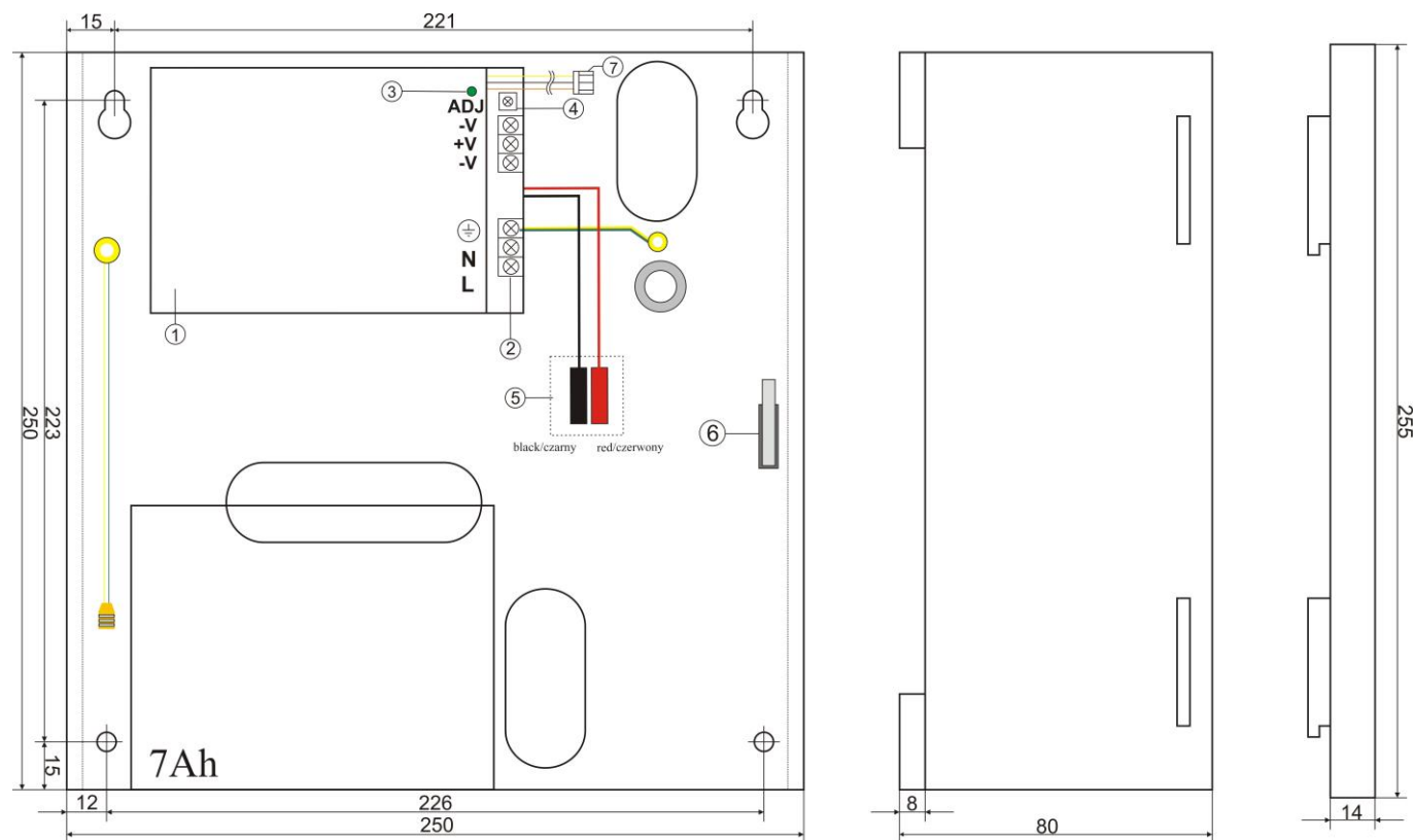
Rys.2. Widok zasilacza.
