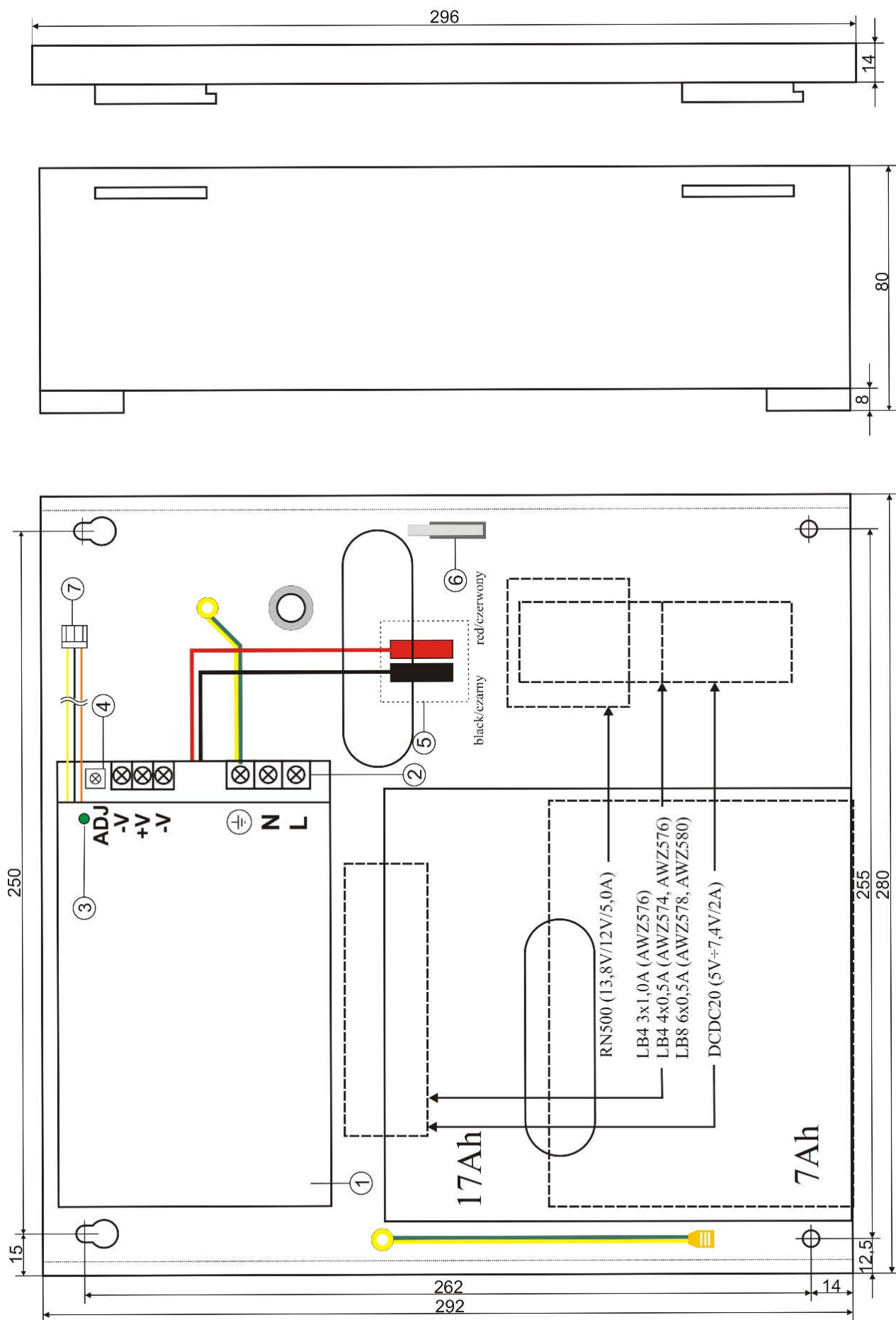
Rys.2. Widok zasilacza.
