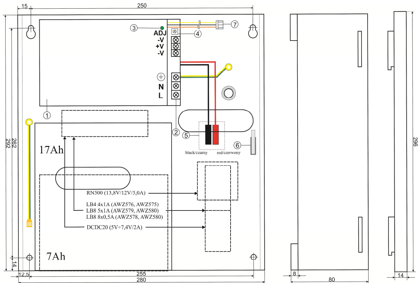
Rys.2. Widok zasilacza.
