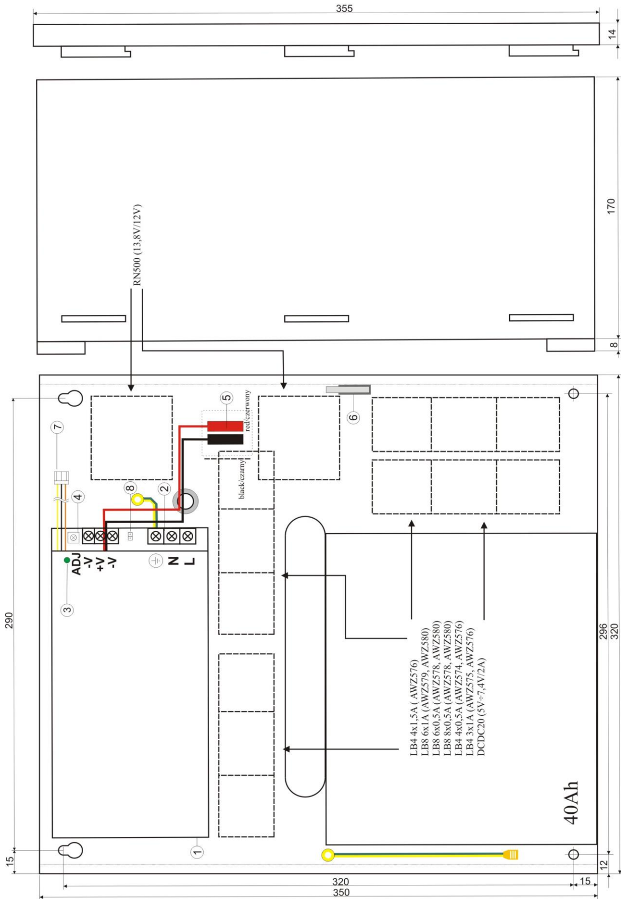
Rys.2. Widok zasilacza.
