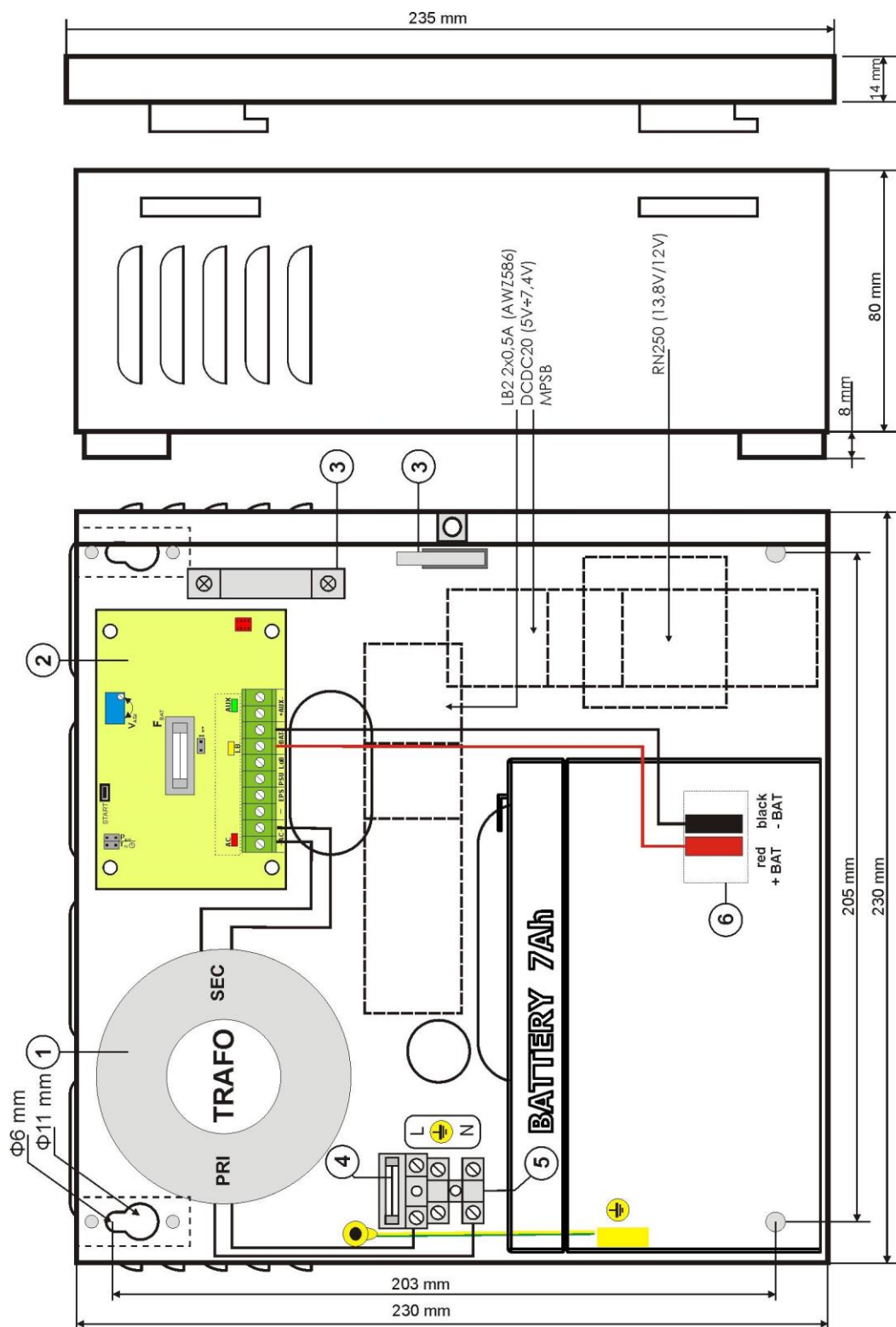
Rys.3. Widok zasilacza.
