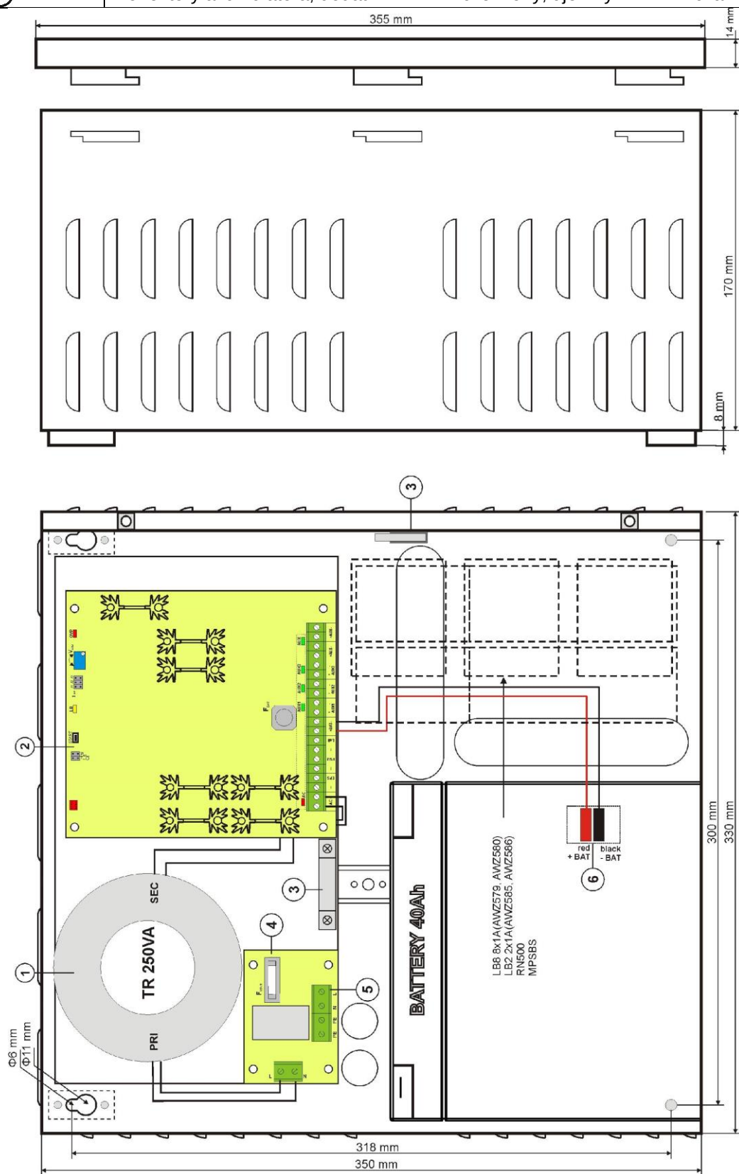
Rys.3. Widok zasilacza.
