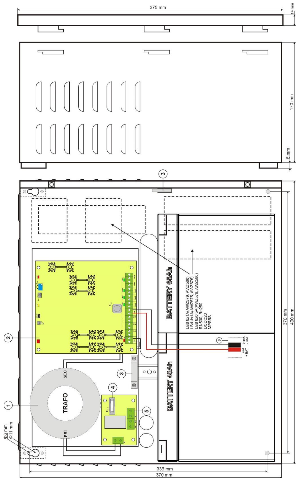
Rys.3. Widok zasilacza.
