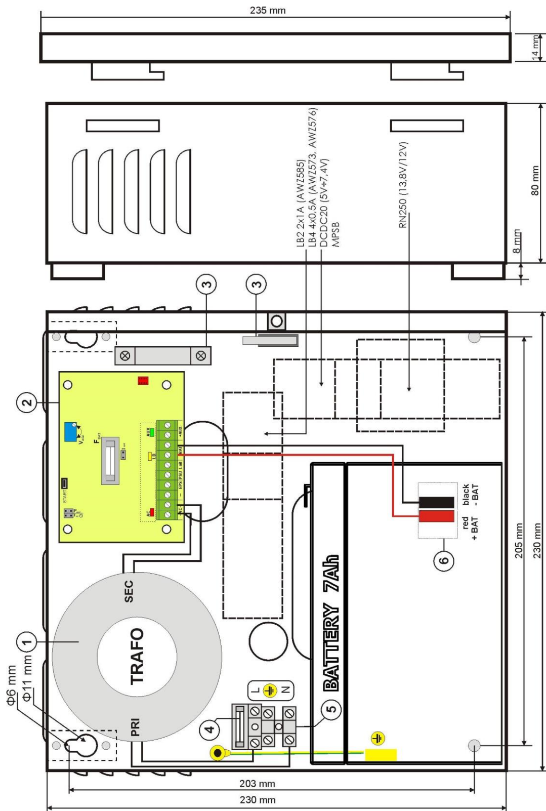
Rys.3. Widok zasilacza.
