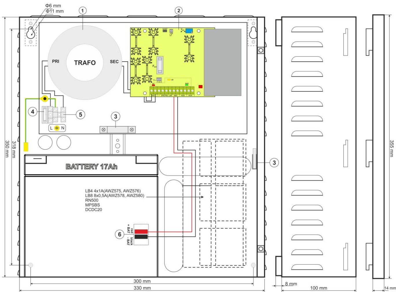
Rys.3. Widok zasilacza.
