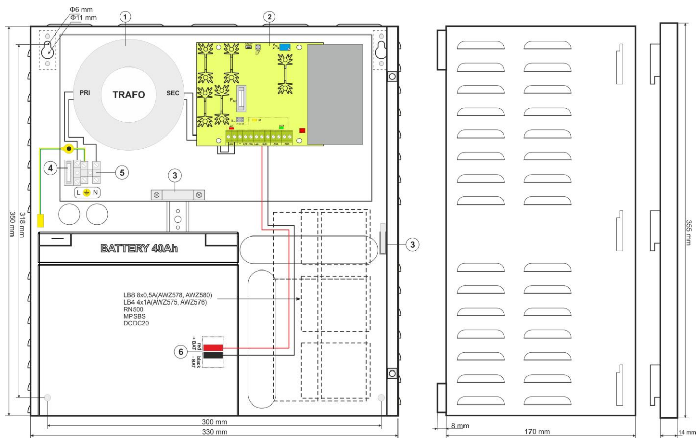
Rys.3. Widok zasilacza.
