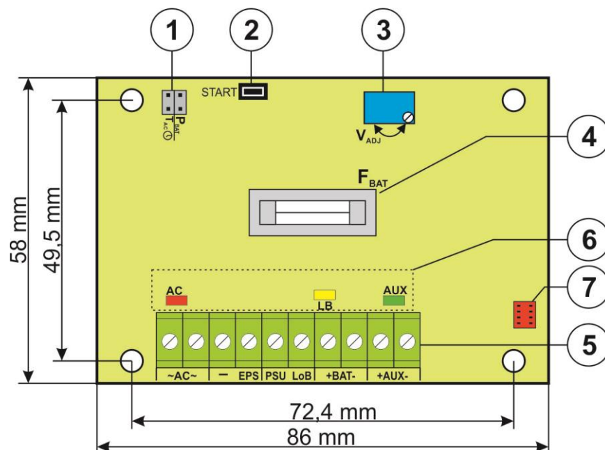
Rys. 2. Widok płyty pcb zasilacza.
