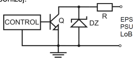
Rys. 4. Schemat elektryczny wyjść technicznych OC.
