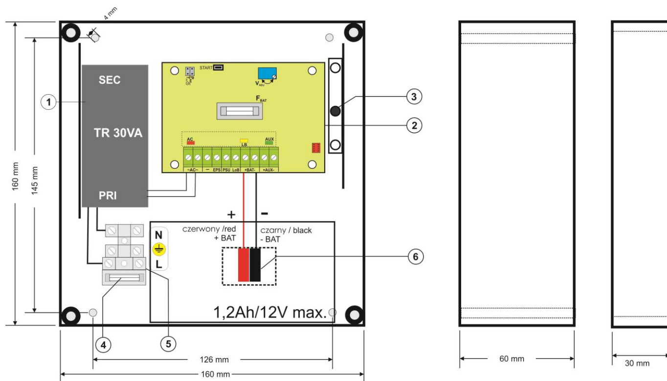
Rys.3. Widok zasilacza.
